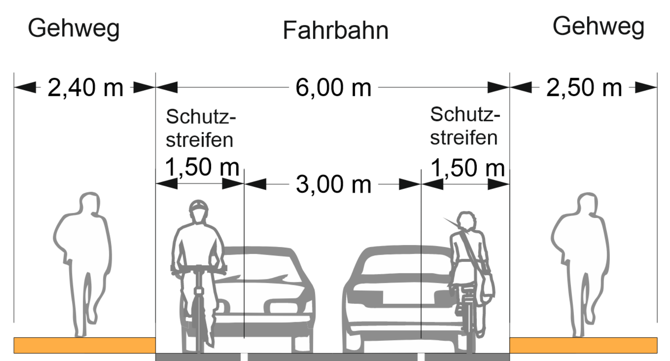
Querschnitt 2
