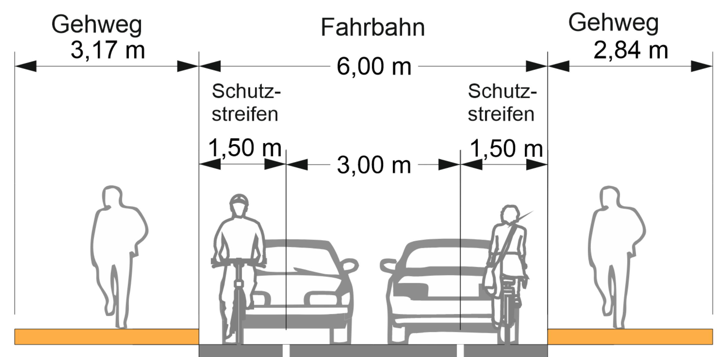
Querschnitt 1
