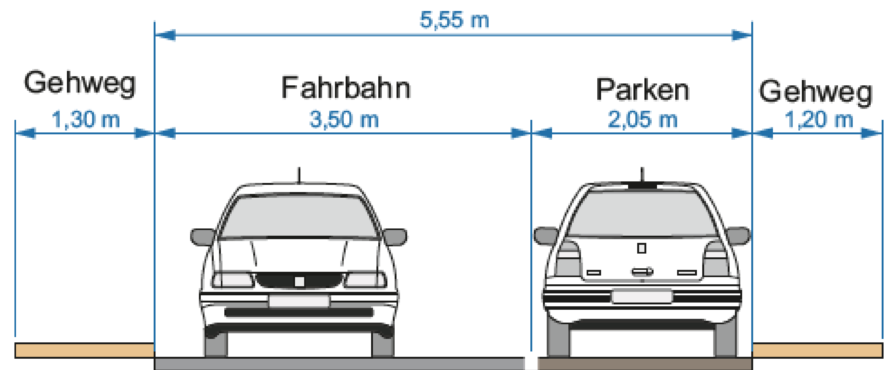
Querschnitt 6
