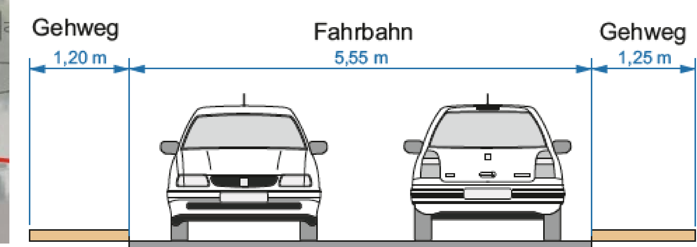
Querschnitt 7
